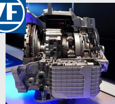
ZF 9HP 9AT Transmission
