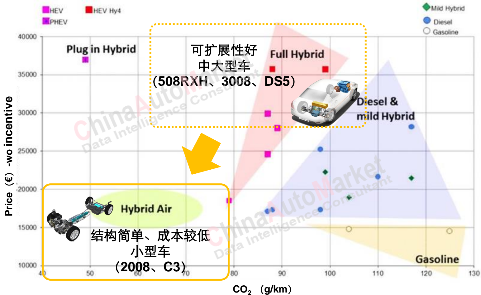
Hybrid Air系统与其他混合动力系统成本及减排效果对比
